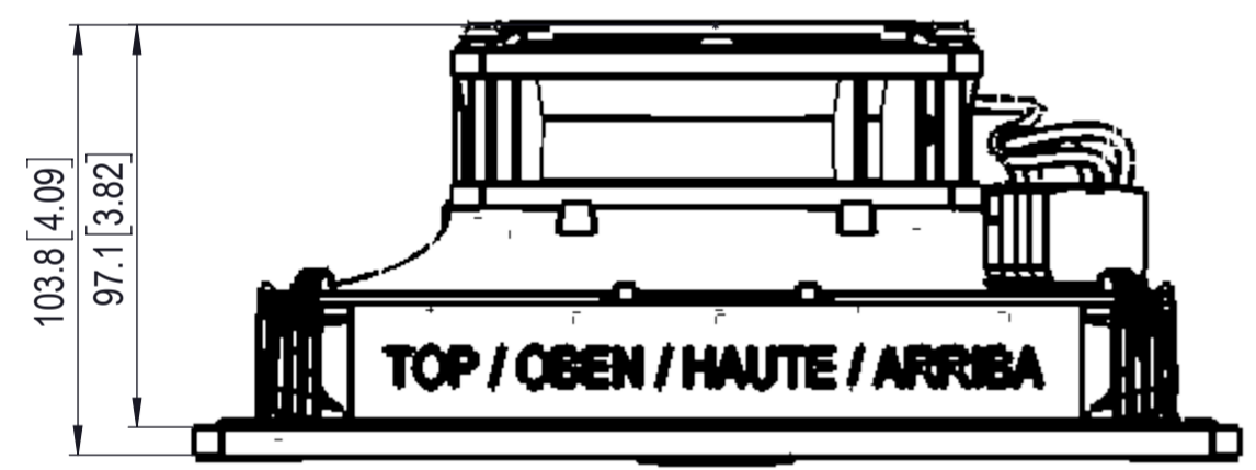
B-B view without / Absicht ohne Pos. 1,2,8
